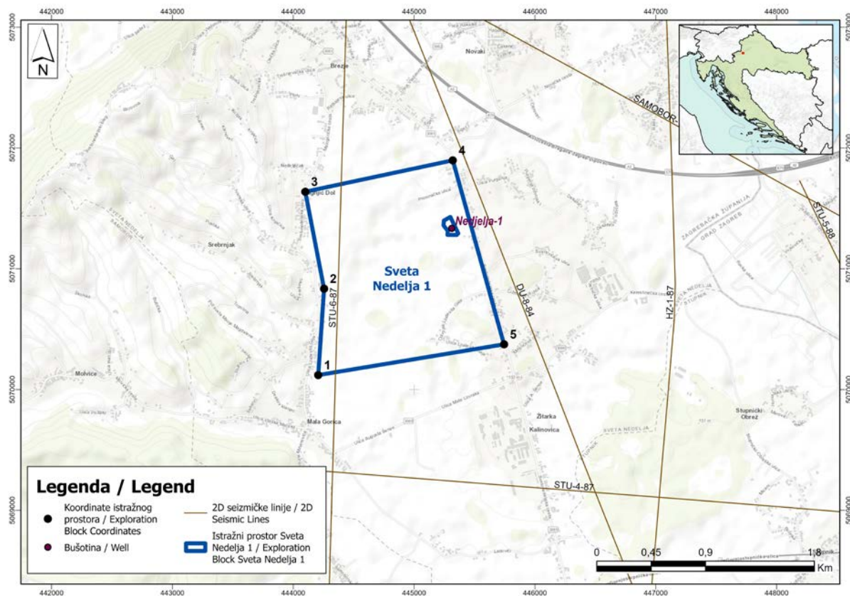
Slika 4. Podaci dostupni na istražnom prostoru „Sveta Nedelja 1“
