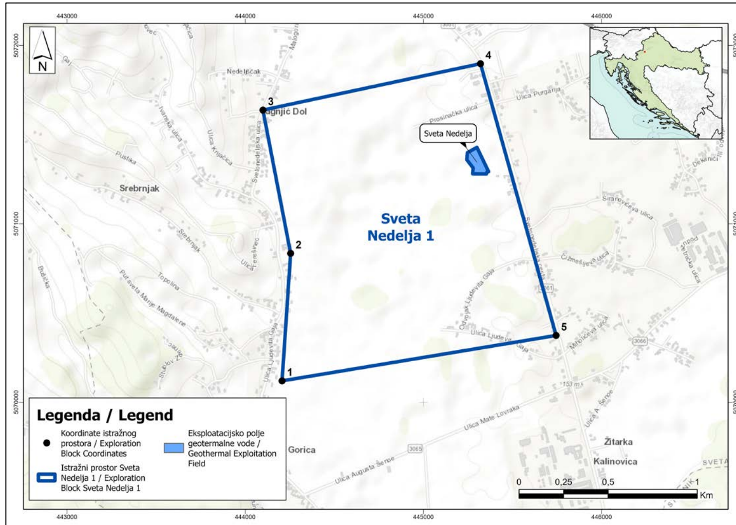
Slika 1. Pregledni zemljovid istražnog prostora „Sveta Nedelja 1“
